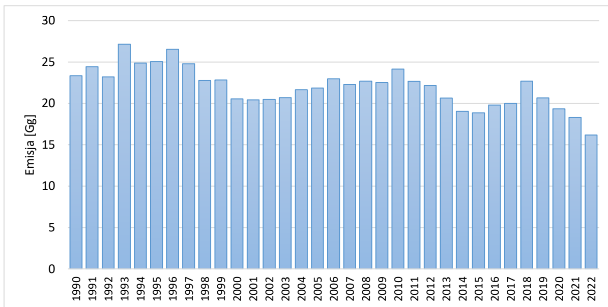
Rysunek 18. Trend emisji BC (sady) w latach 1990 – 2022
