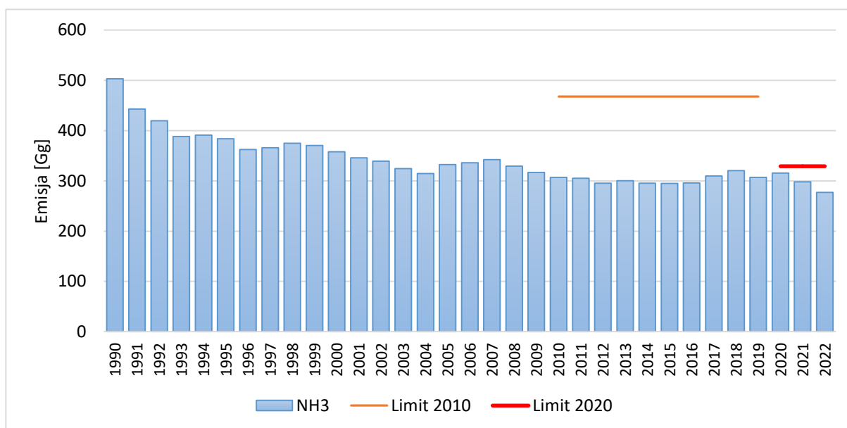
Rysunek 8. Trend emisji \text{NH}_3 w latach 1990-2022
